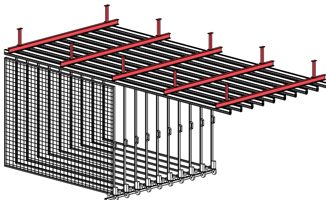
Befestigung an die Decke mit abgehängter Stahlkonstruktion
